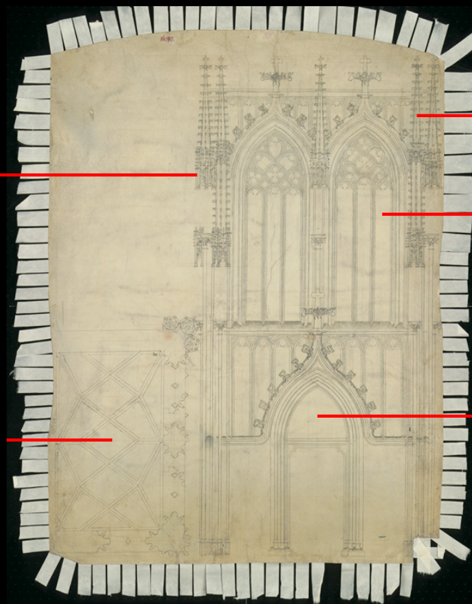
Aufriss- und Grundrisszeichnung der Vorhalle der Maria-Magdalena-Kapelle.
