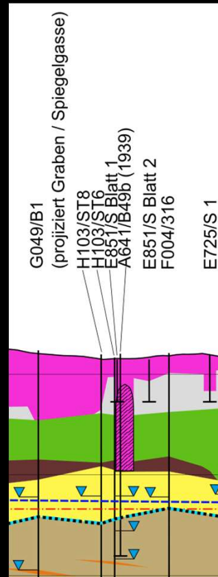
Hydrogeologischer Längenschnitt
